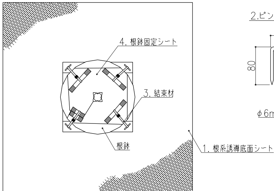
施工平面図 S=1:10
