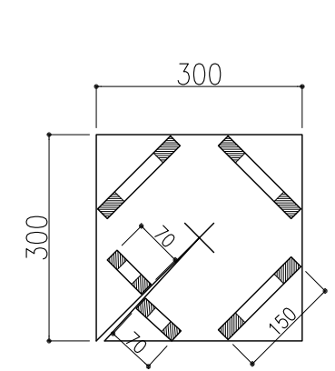
4.根鉢固定シート S=1:10
