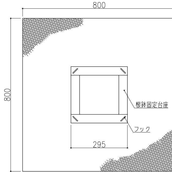
1.根系誘導底面シート S=1:10
