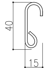
5.補助ロープフック S=1:2
