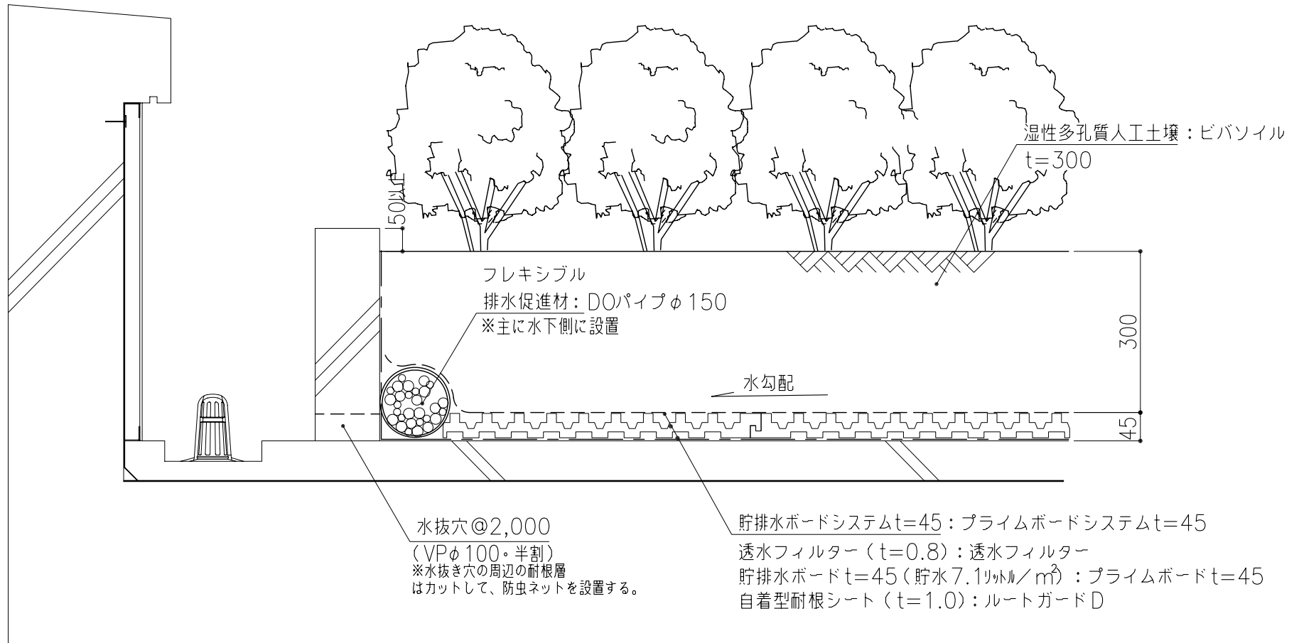
ビバソイルシステム 断面詳細図
