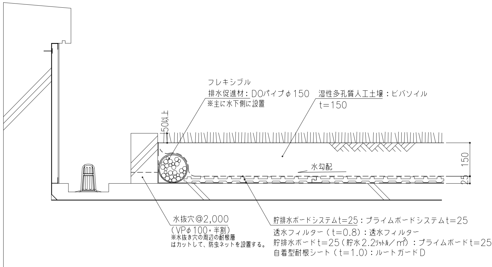
ビバソイルシステム 断面詳細図
