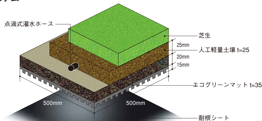
システム断面図 ※自動灌水システムは標準装備です。
